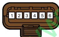
D24 右后门门锁电机
