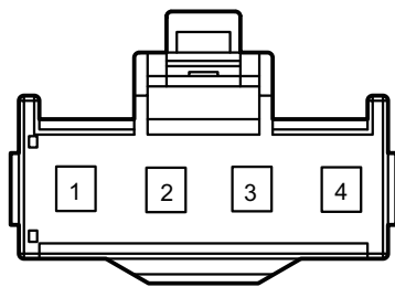
X05 发动机舱线束接仪表线束B（母端）
