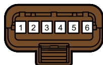
D16 左后门门锁电机
