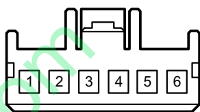
S48 后背门门锁电机
