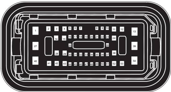
X21 底盘线束接左前门线束（公端）
